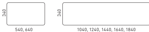
Zusammensetzung der Plexiglas (Perspex) Knieblende
